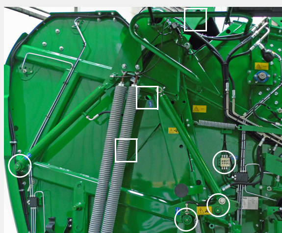
Voitelupisteet NDS (Ei ajon puoli)
