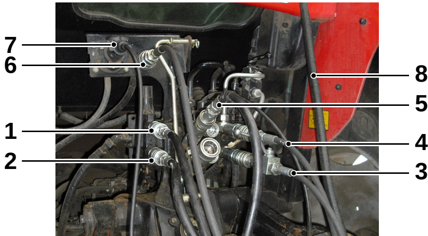
Hydrauliletkujen ja sähköjohdinten mahdollinen asetelma
