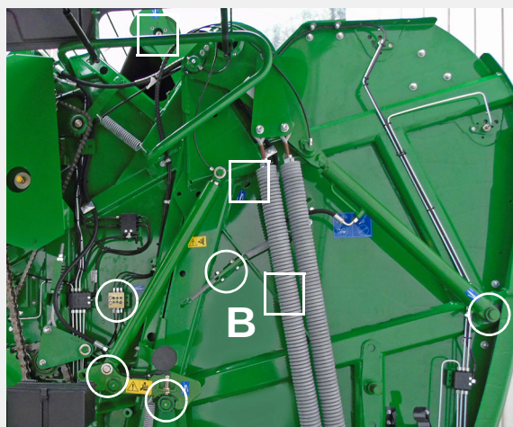
Voitelupisteet DS (ajon puoli)
