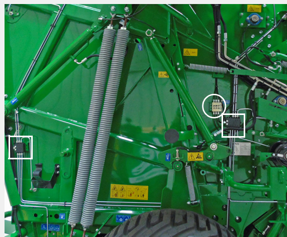
Voitelulohkot NDS (ei ajopuoli)
