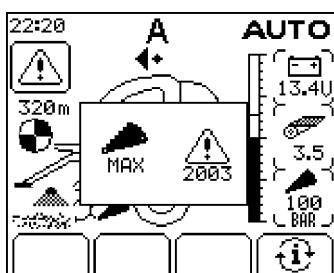
Teräpaine on liian korkea -varoitus
