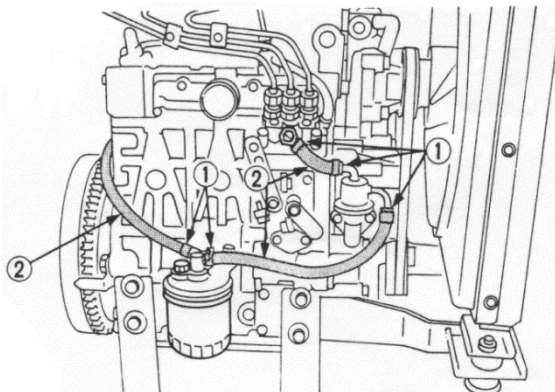
2) Polttoaineletkut
