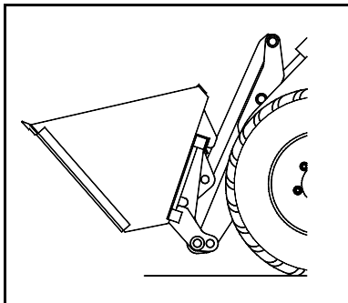
Kuva 1 Työkalun kiinnittäminen
