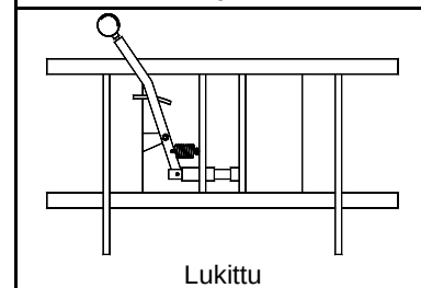
Kuva 2 Työkalun lukitseminen
