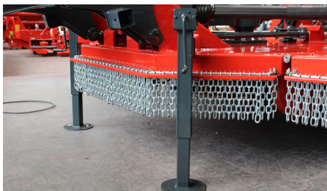
Kaksi kestävää tunkattavaa tukijalkaa. Työn ja kuljetuksen ajaksi tukijoi- le on paikka vetoaisassa.
