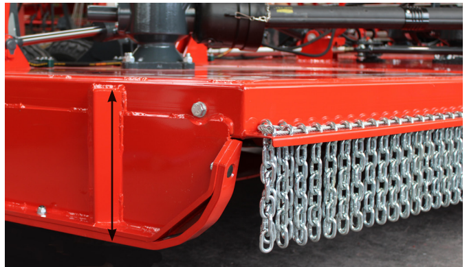
Kannen suuri 33 cm sisäkorkeus mahdollistaa suurten kasvustojen silp- puamisen
