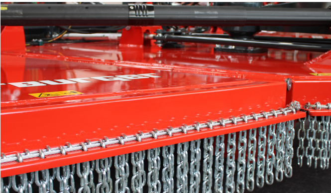
Tasainen kansi vähentää kasvimateriaalin kasautumista ja on helppo pi- tää puhtaana. Kaksoisketjusuojaus on vakiovaruste.
