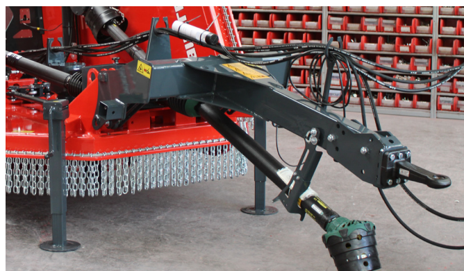
Vetoaisa voidaan kääntää nivelakselin ylä- tai alapuolelle.
