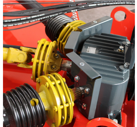
Toisionivelakselit levykytkimellä (2 kitkalevyä)
