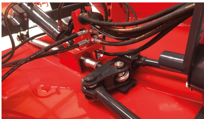
Nerokas säätöjärjestelmä tankojen ja työntövarren yhdistelmänä.
