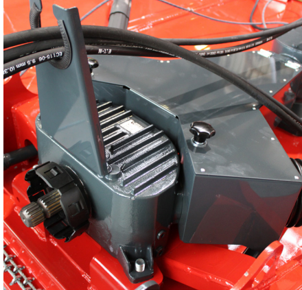
Jakovaihteisto huohottimella - tehonkesto 290 hv - öljytilavuus 3,8 l
