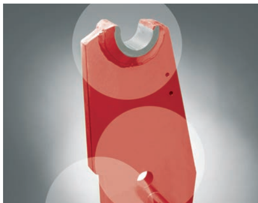
Yksinkertainen ja kestävä Delta-sovite, jossa kolme kontaktipistettä
