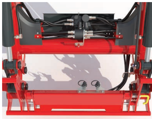
Poikkiputki sisältää hydraulikomponentteja ja vahvistaa rakennetta heikentämättä näkyvyyttä
