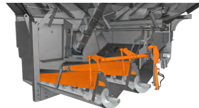
▲ Säädettävä tyhjennysnopeus
