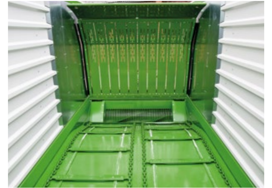
Kallistettu pohjakuljetin, 4 ketjua (14 x 50 mm, 25 tn/ketju)
