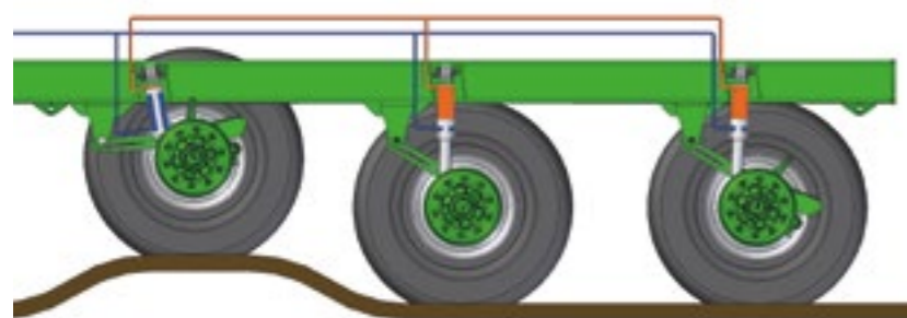
Teli and kolmeakselinen hydraulisella rungolla
