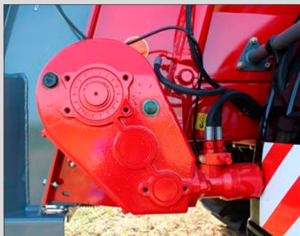
Pohjakuljettimen hydrauliimoottori ja raskaalle käytölle suunniteltu vaihteisto
