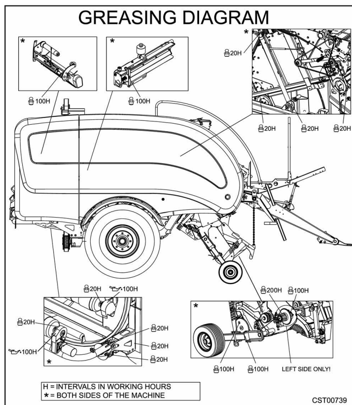
Rasvauskaavio
