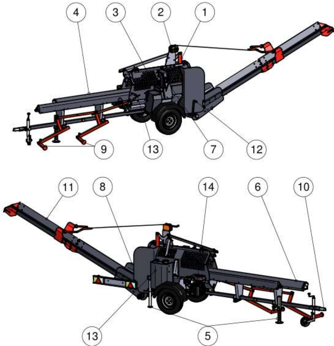
Kuva 1. Pilkekoneen pääosat
