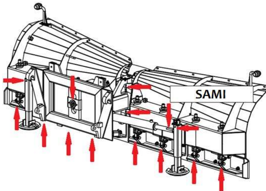
Piirros 4. Voitelunippojen paikat
