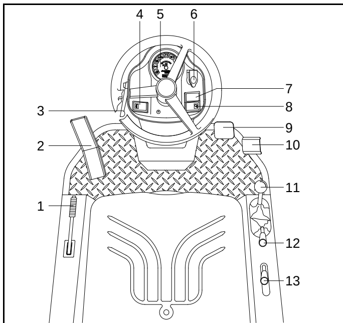
1. Seisontajarrun vipu
