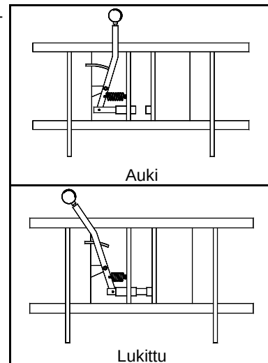
Kuva 2 Työkalun lukitseminen
